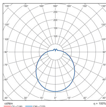
BRS-B 27W 4000°K:
