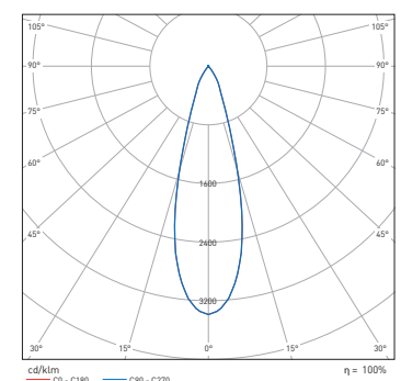
Dragon 3000°K 30°:
