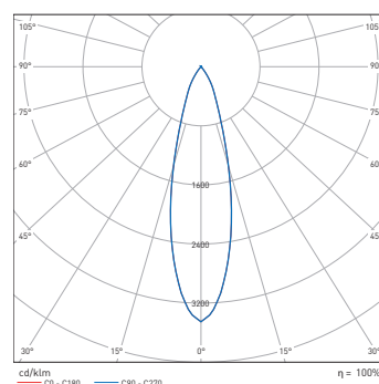
Dragon 3000°K 30°:
