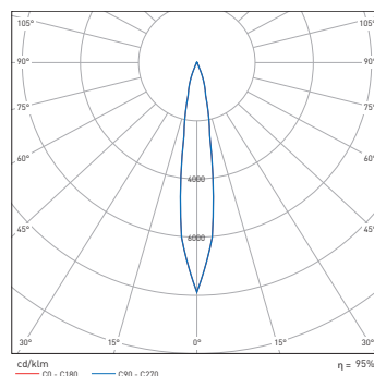
DINO mit Reflektor 3000°K 15°:
